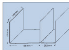
Kanisterstütze aus Aluminium für sicheren Stand
