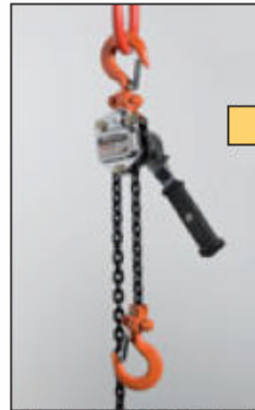
Hebelzug Mini, 250 kg Traglast, Bestell-Nr. 179-269
