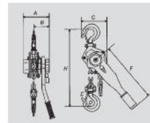
Hebelzug Standard, ab 750 kg Tragkraft
