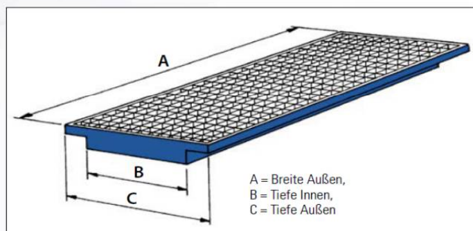
Regalwanne Typ SRW aus Stahl
